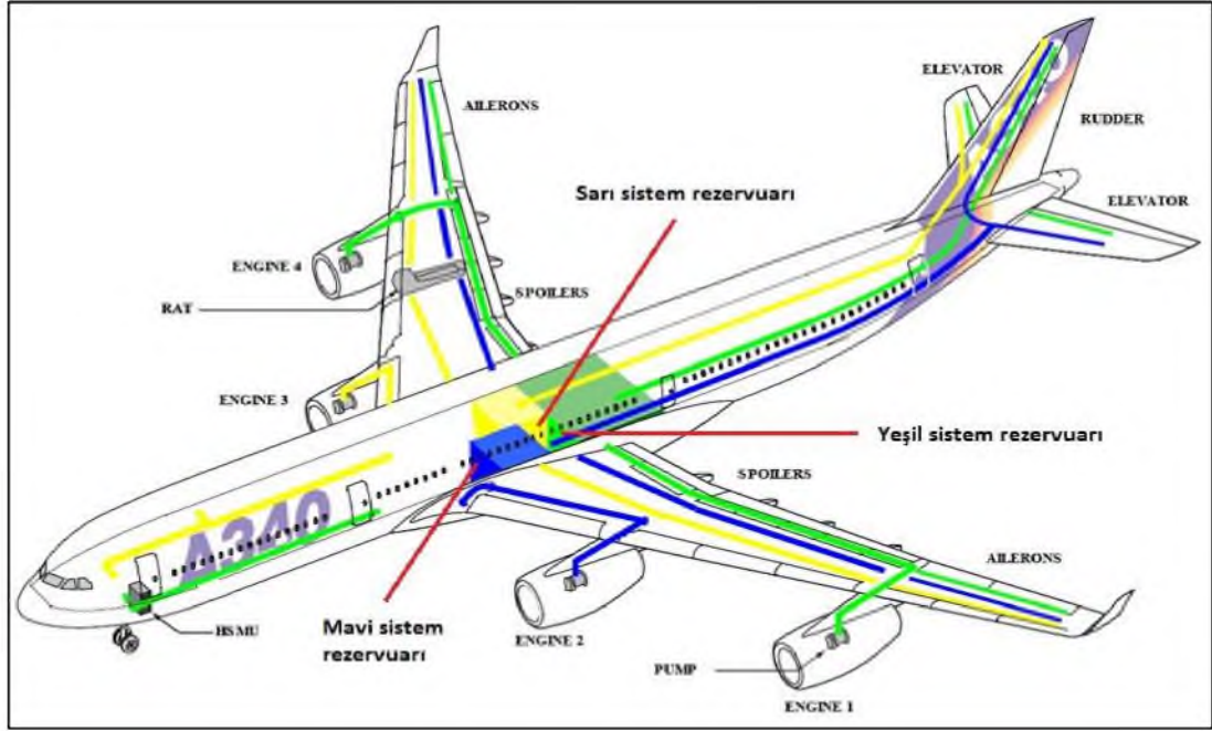
Şekil 15: Airbus A 340 uçağındaki hidrolik sistemlerin beslediği ekipmanlar
