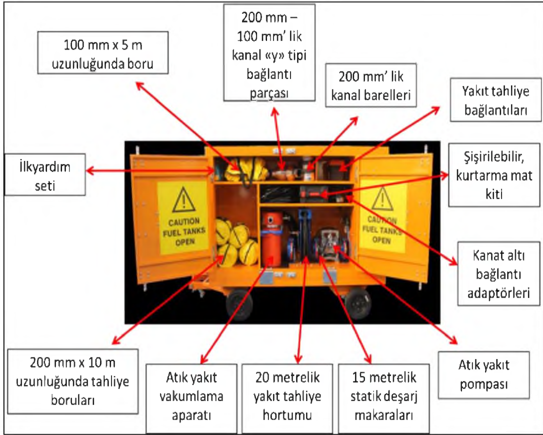
Resim 62: Purge air sisteme ait konteynırın sol kısmında yer alan ekipmanlar (THY Teknik A.Ş. teknik eğitim dokümanları)
