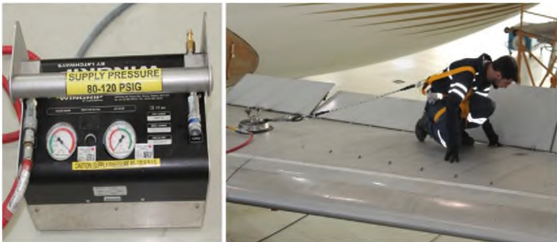
Resim 26: Çapalara giden havanın basıncını ayarlayan wingrip regülatörü
