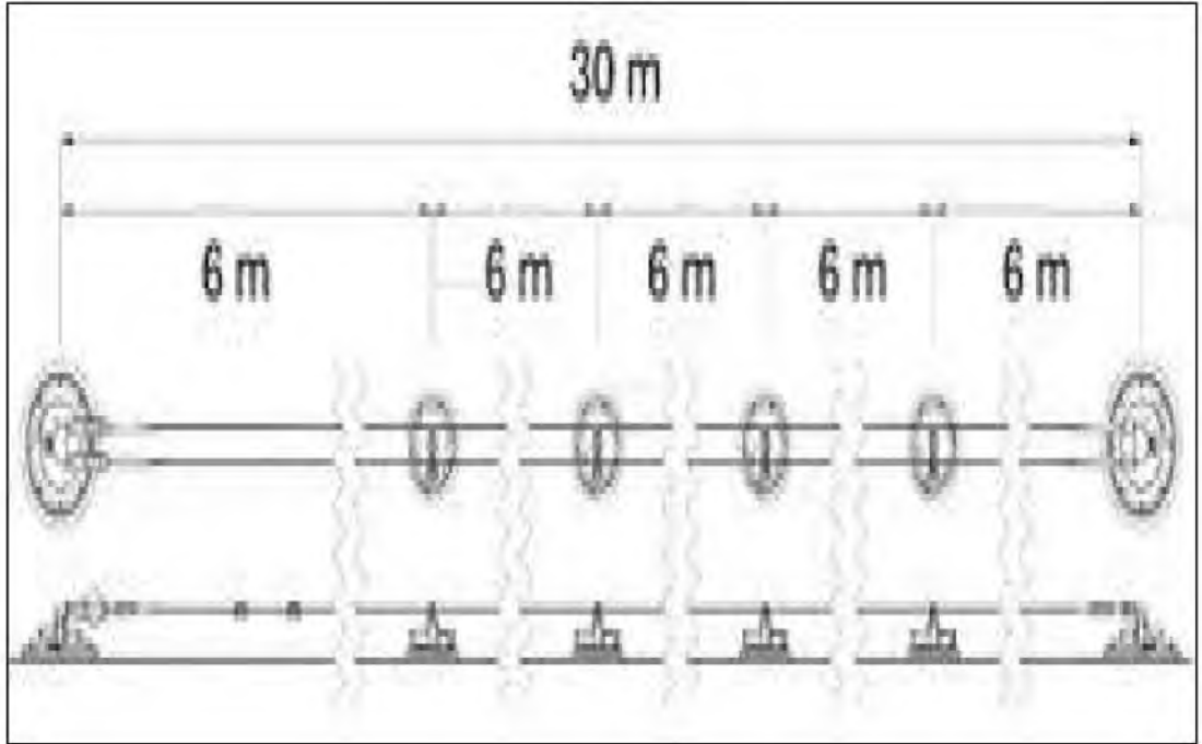
Şekil 7: Bir wingrip ikiz hat sisteminin tipik düzeni
