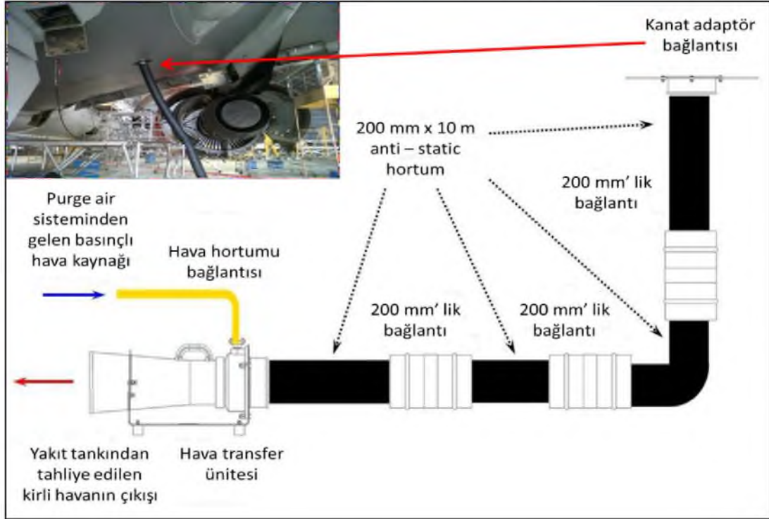
Resim 65: Purge air sistemin yakıt tankı ç çalışmalarındaki uygulamasına bir örnek (THY Teknik A.Ş. teknik eğitim dokümanları)
