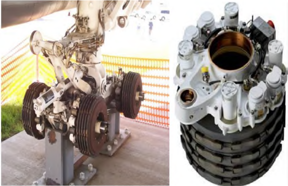
Resim 54: Uçak brakeunitleri (fren ünitesi)
