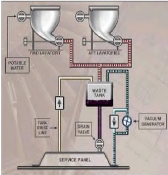
Şekil 13: Waste hattı
