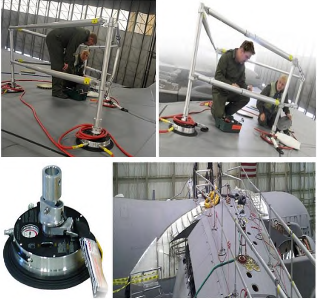
Resim 27: Wingrip korkuluk ve bariyer sistemi
