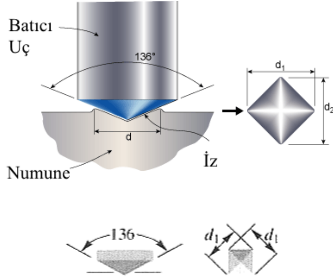
Şekil 10.2: Vickers sertlik deneyi
