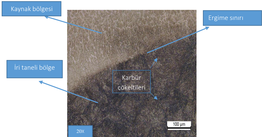
Şekil 12.11: HARDCOR 600G TEK PASO Numunesinin ITAB Görüntüsü Görüntüsü (20X)
