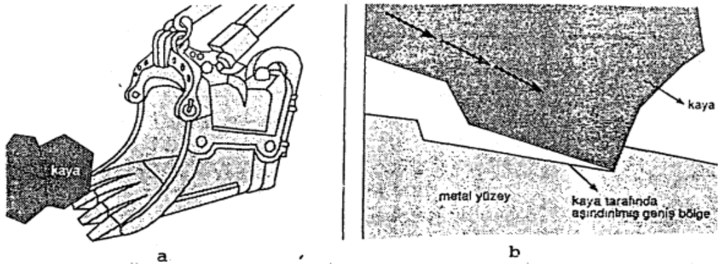
Şekil 9.5: (a) Düşük Hız ve Kuvvetle Kaya Ağırlığının Metale Darbesi ve Kayanın Metal Yüzeyi Oyararak Aşındırması, (b) Şematik Görüntüsü (Mustafa Aydın 1996)
