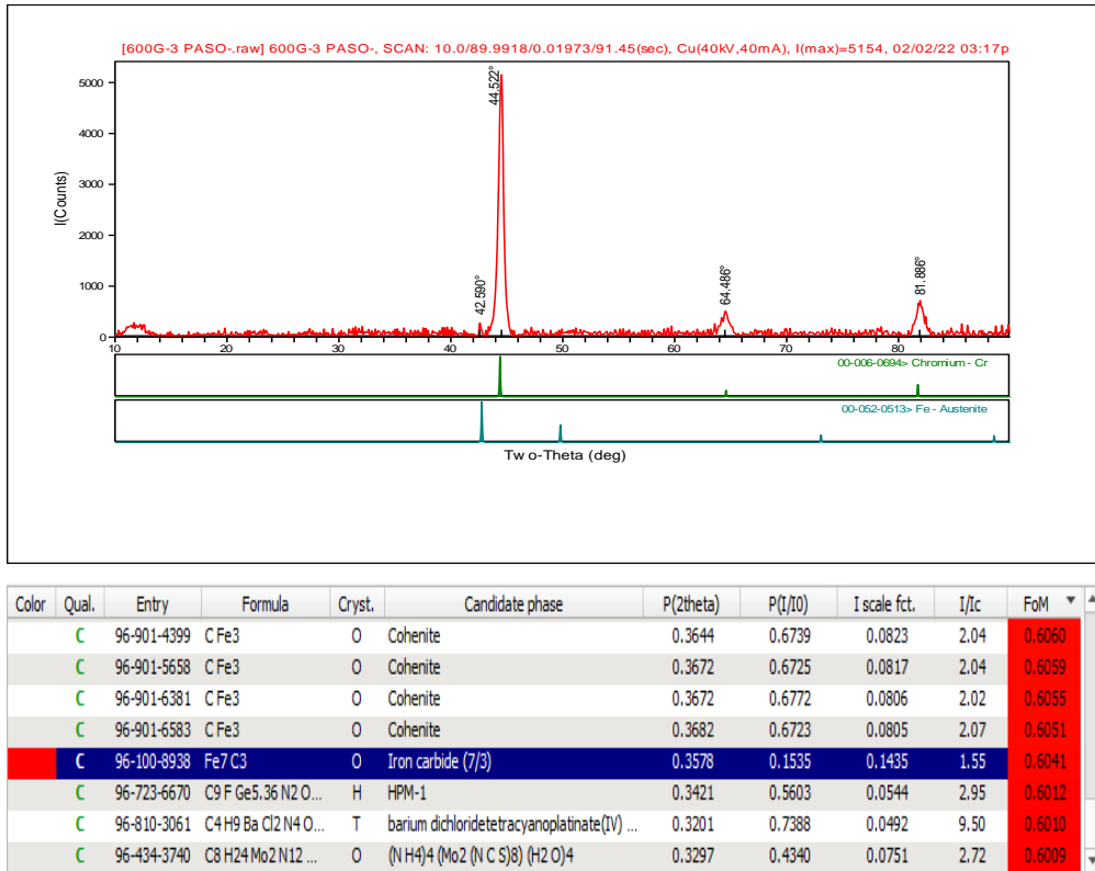
Şekil 12.17: HARDCOR 600G 3 Paso XRD Analizi Görüntüsü
