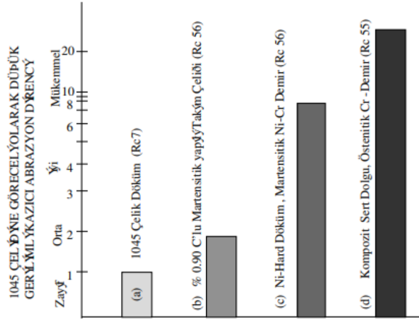
Şekil 8.1: Aşınma Direncinin Sertlik ile Karşılaştırılması
