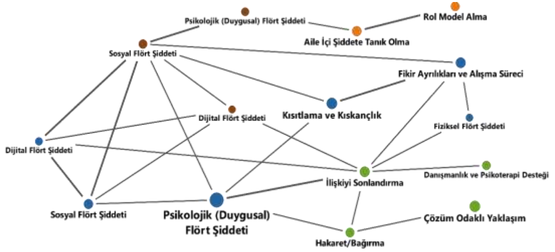
Şekil 4.10: Kod Haritası
