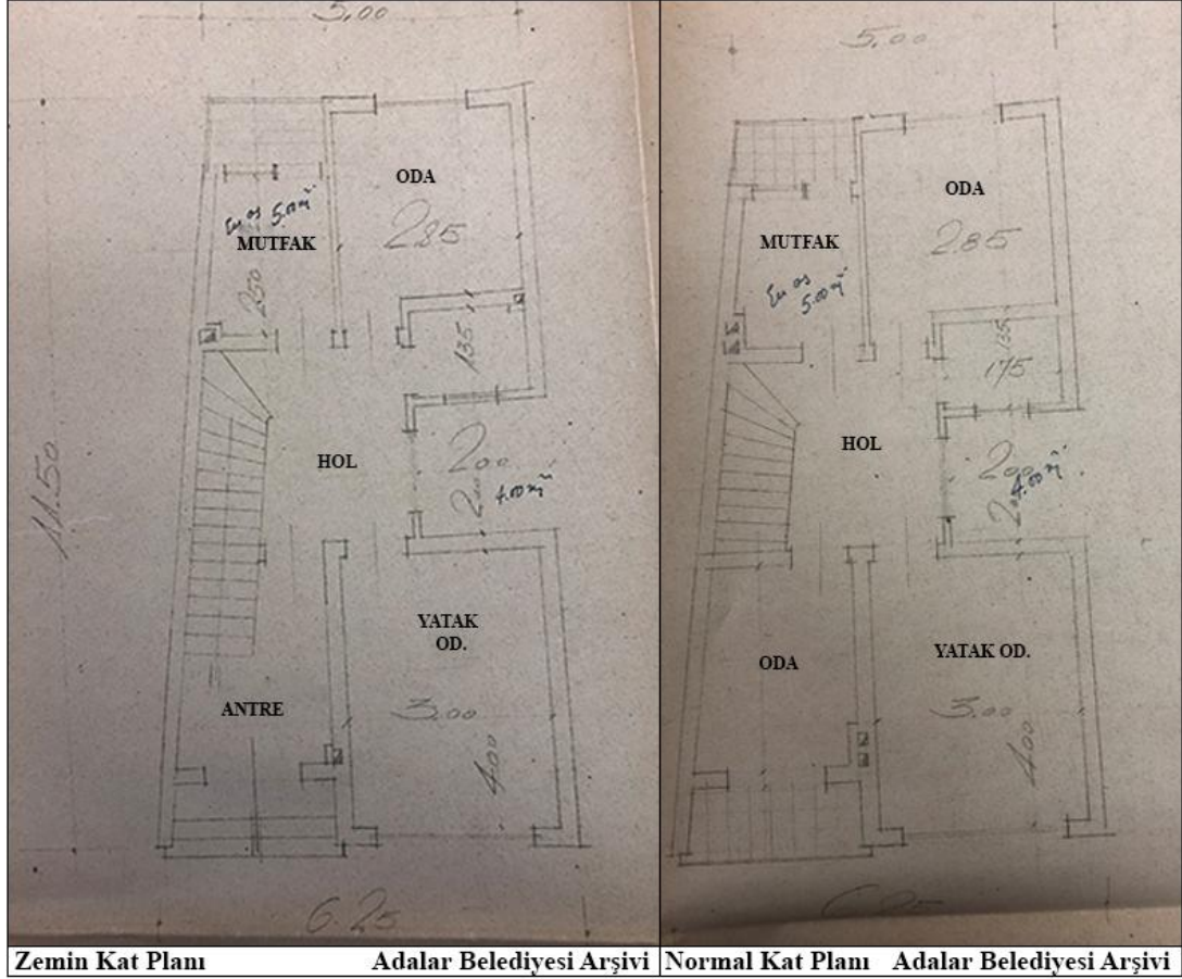
Şekil 4.19: Çavuşođlu Köşkü-II'ye ait plan çizimleri
