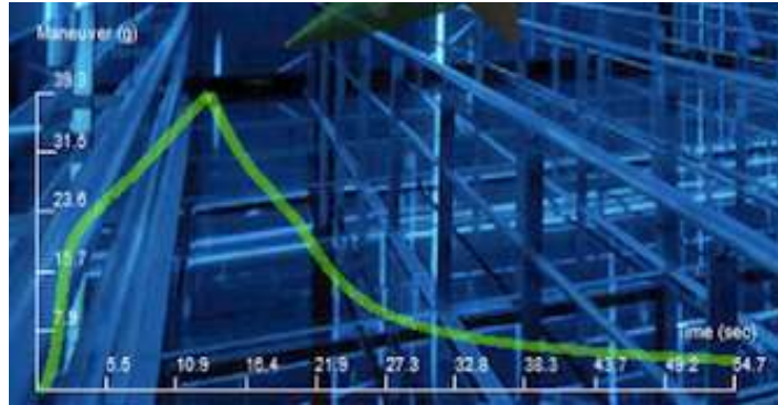
Şekil 4.58: Low Drag_8 Füznesinin Statik Test Manevra Deđeri
