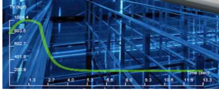
Şekil 4.31: Low Drag_8 Füzesinin Roket Motorunun İtki Kuvveti
