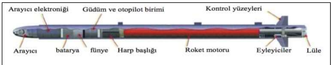
Şekil 2.7: Louyang PL-10 tipi Havadan Havaya Füzede Alt Sistemlerin Yerleşimi
