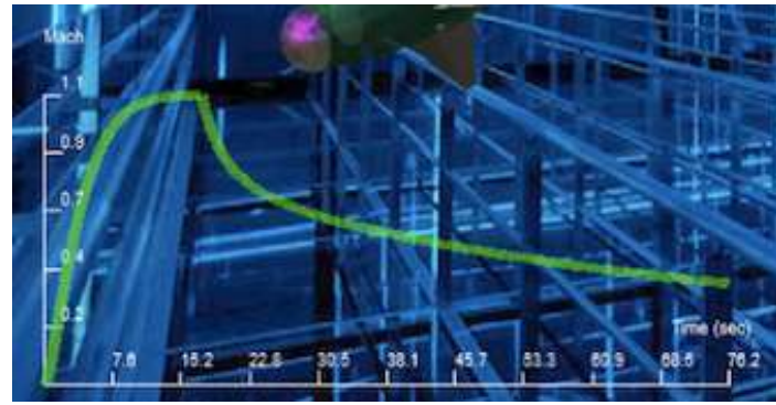
Şekil 4.28: Atgm_1 Füzesinin Statik Test Mach Sayısı
