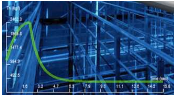
Şekil 4.60: Patriot_TR Füzesinin Roket Motorunun İtici Kuvveti
