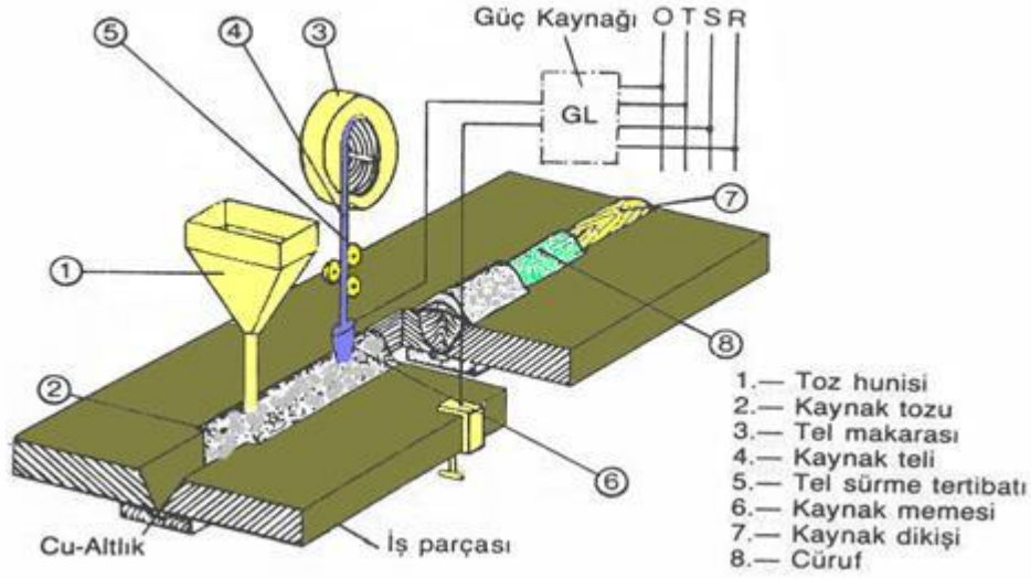
Şekil 4. 4: Tozaltı Kaynak Prensibi (URL-13, 2021)
