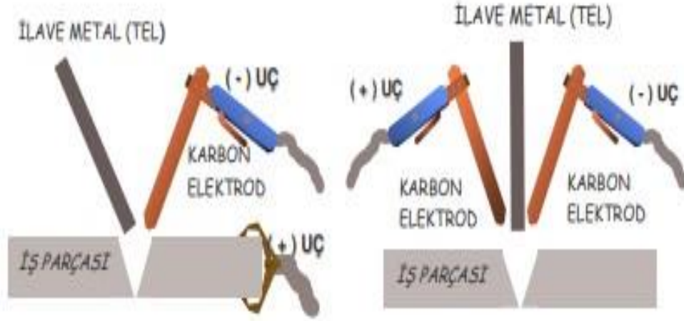
Şekil 2. 4: Karbon Arkı İle Yapılan Birleştirme Amaçlı Kaynak Uygulamaları (Erkan, K. 2014)
