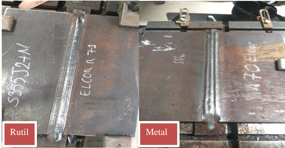
Şekil 9. 1: Rutil ve Metal Özlü Tel Kaynak Numunelerinin Fotoğrafları
