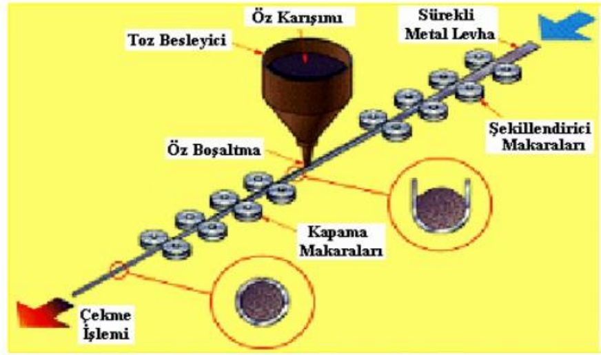
Şekil 6. 2: Öz­lü Telin Üretim Detayı (GEV, IIW No:1.8.2, 2012)
