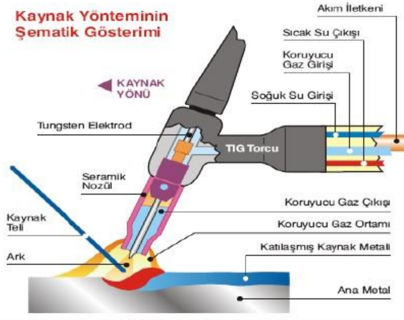
Şekil 5. 7: TIG Kaynak Torcunun Şematik Gösterimi (URL-19, 2021)
