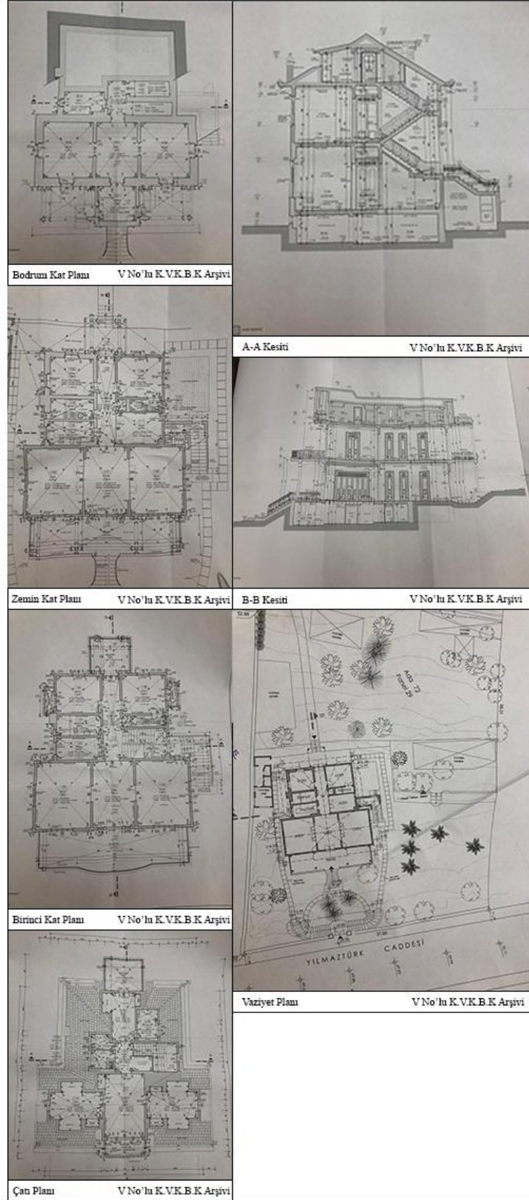
Şekil 4.14: Usulcuoğlu Köşkü-II'ye ait plan ve kesit çizimleri
